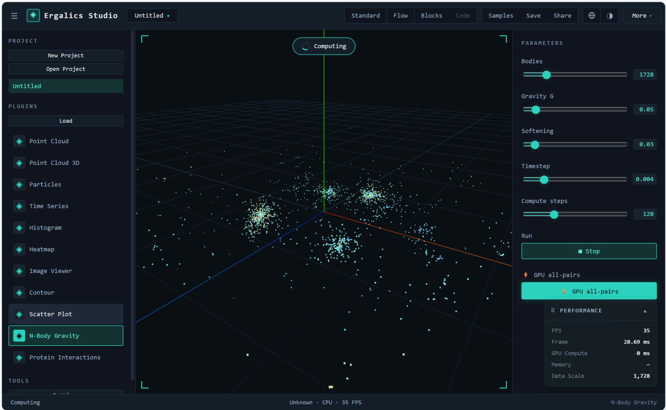
N-Body 引力
